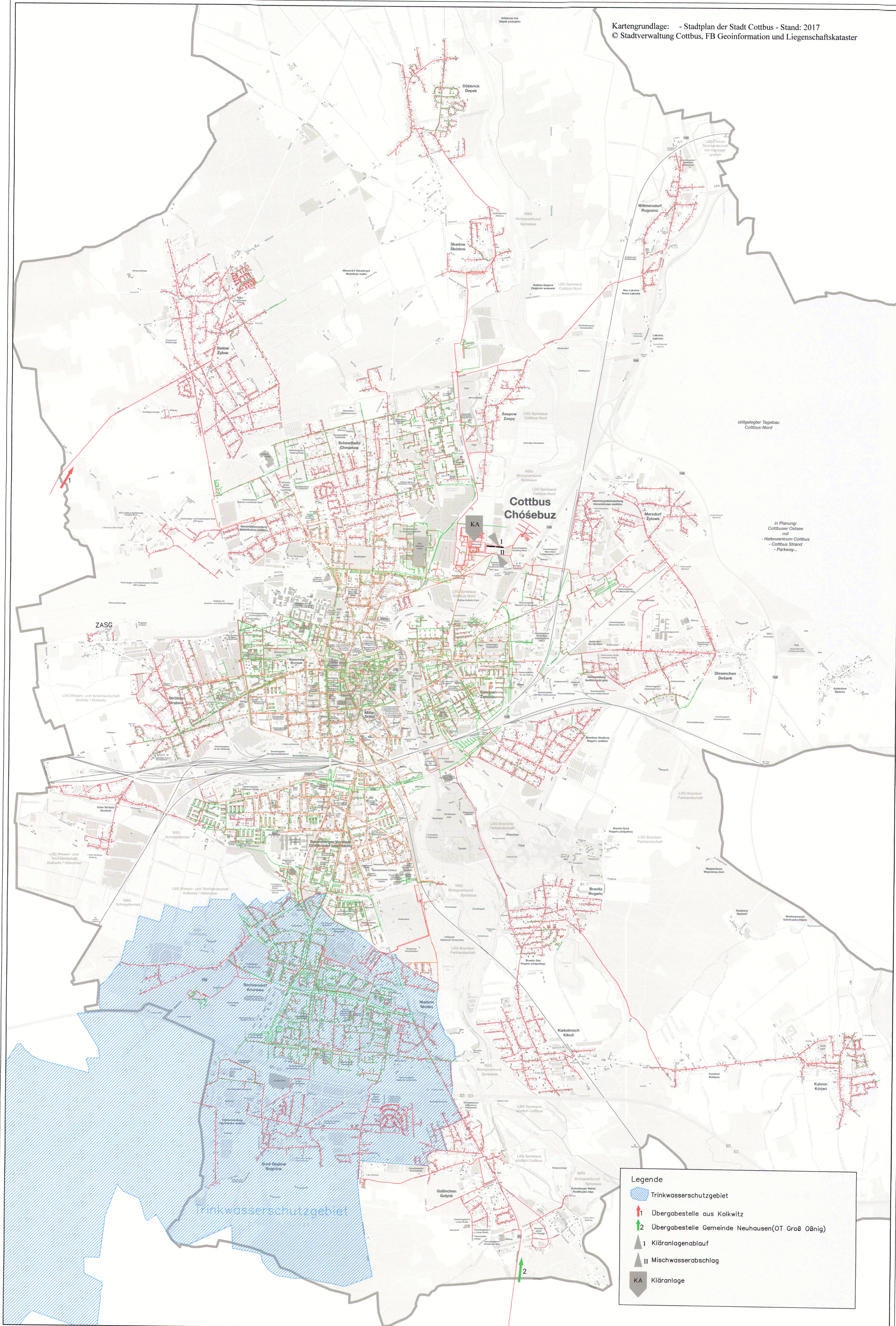
Abwasserbeseitigungskonzept der Stadt Cottbus – Ergänzung Oktober 2019 (Nachtrag für OT Kiebusch) Übersichtsplan Abwasserentsorgungssystem
