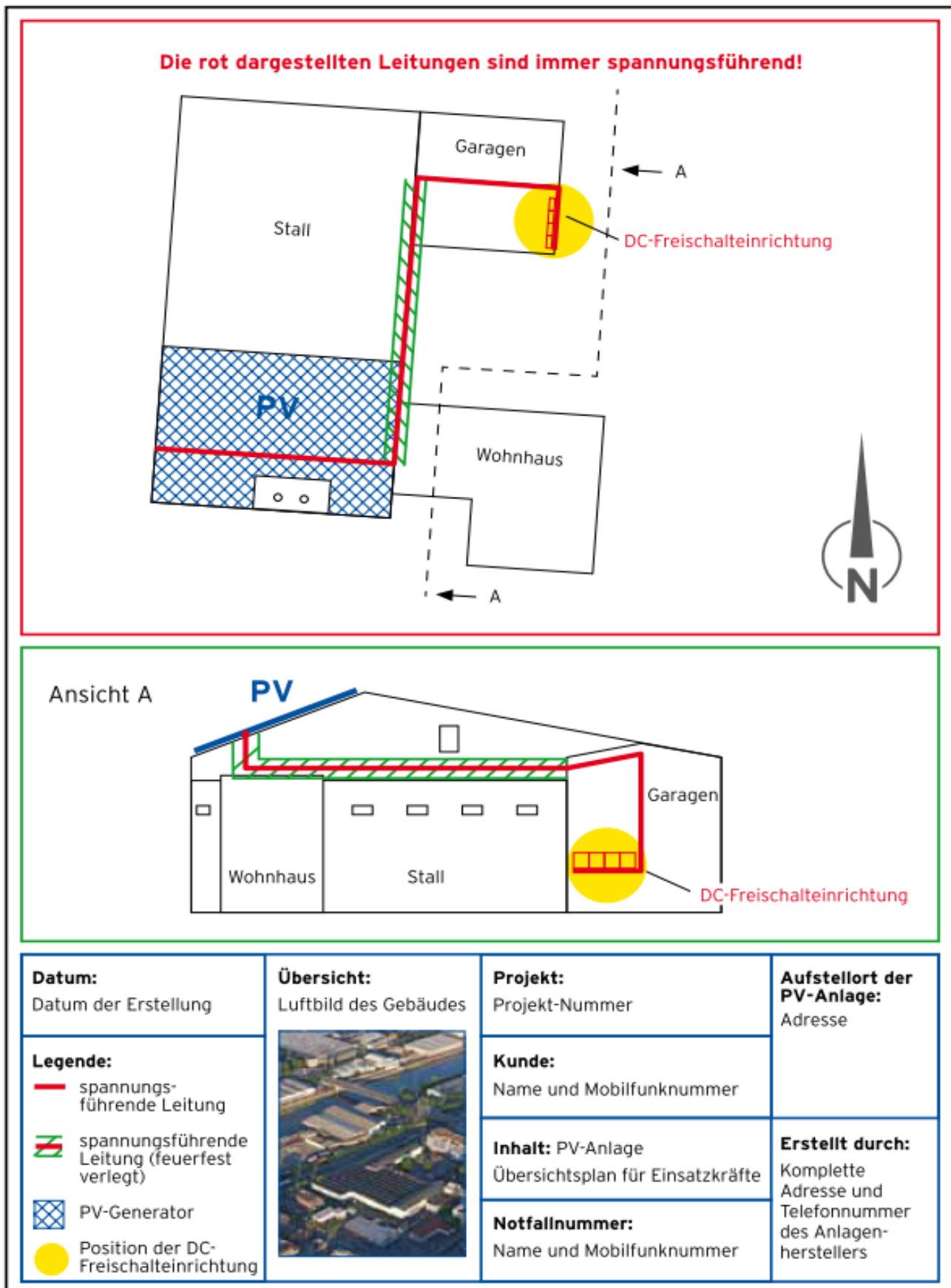
Vorlage 3: Muster eines Übersichtsplanes für Einsatzkräfte nach VDE-AR-2100-712
